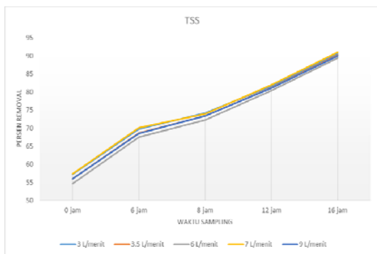
Grafik -2 Hubungan Debit Udara Dan Waktu Sampling Terhadap % Removal TSS
